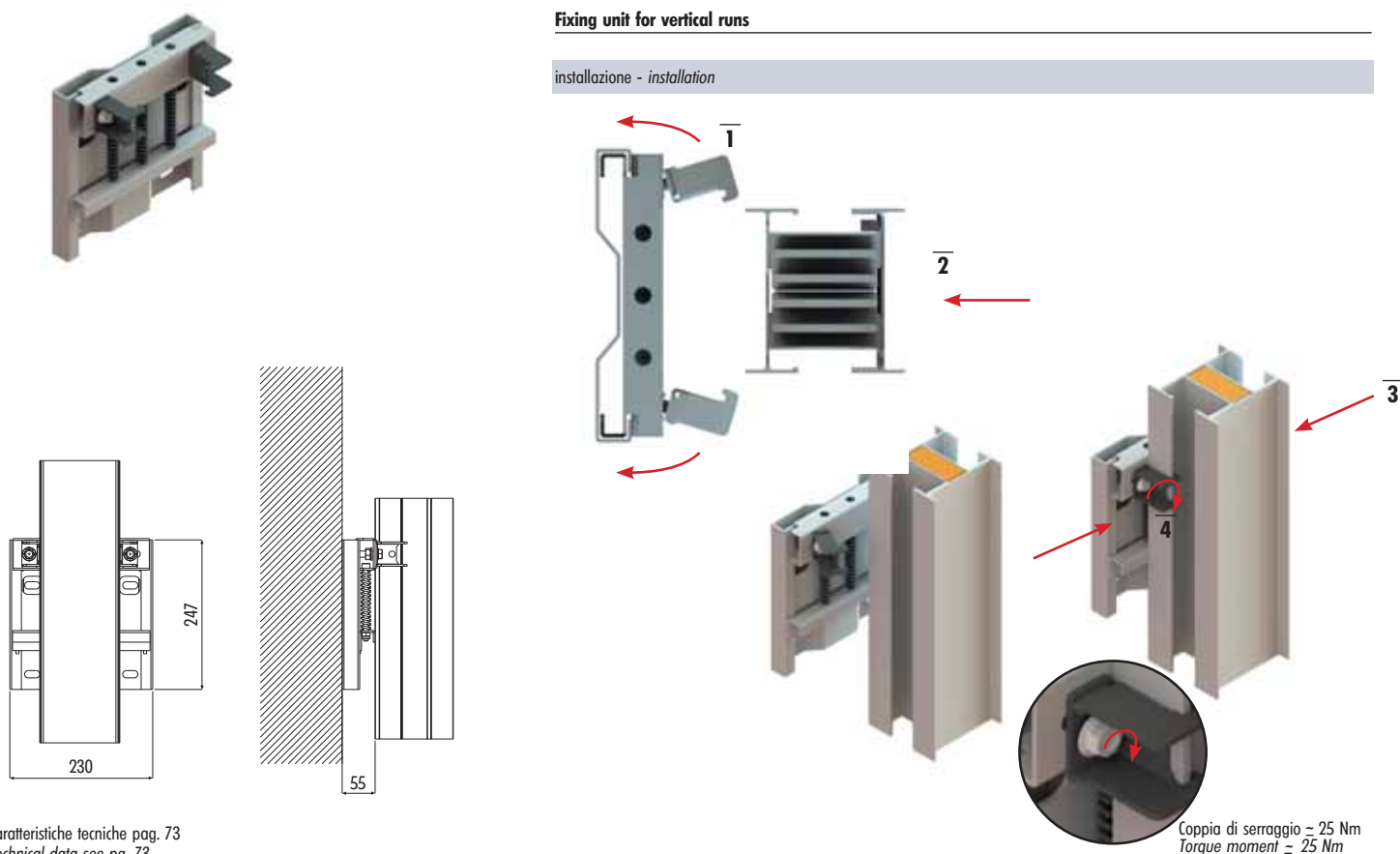
Unità di fissaggio per tratti verticali
